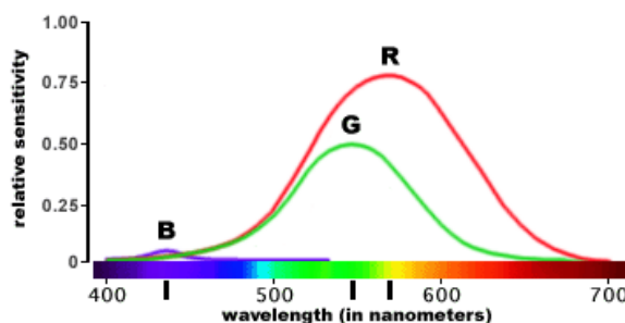
Obr. 7 Citlivost jednotlivých čípků na vlnové délky [39]
