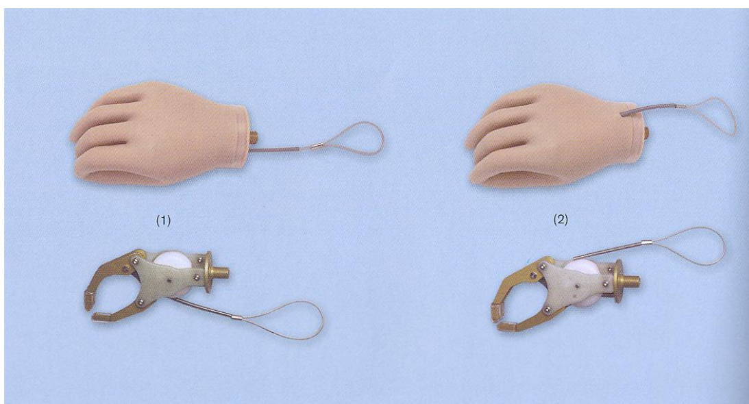
Obr. 25 Vnitřní/vnější tah [30]
