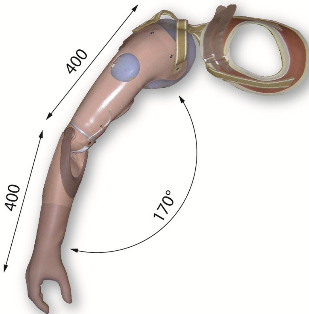
Obr. 64 DynamicArm 12K100 - základní rozměry a rozsahy v extenzi
