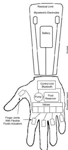
Obr. 40 Struktura hydraulického systému [49]
