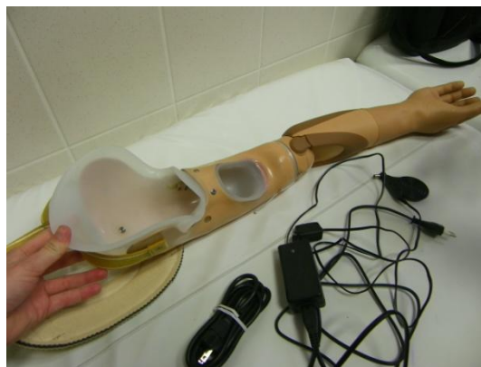
Obr. 61 Hotová pomůcka
