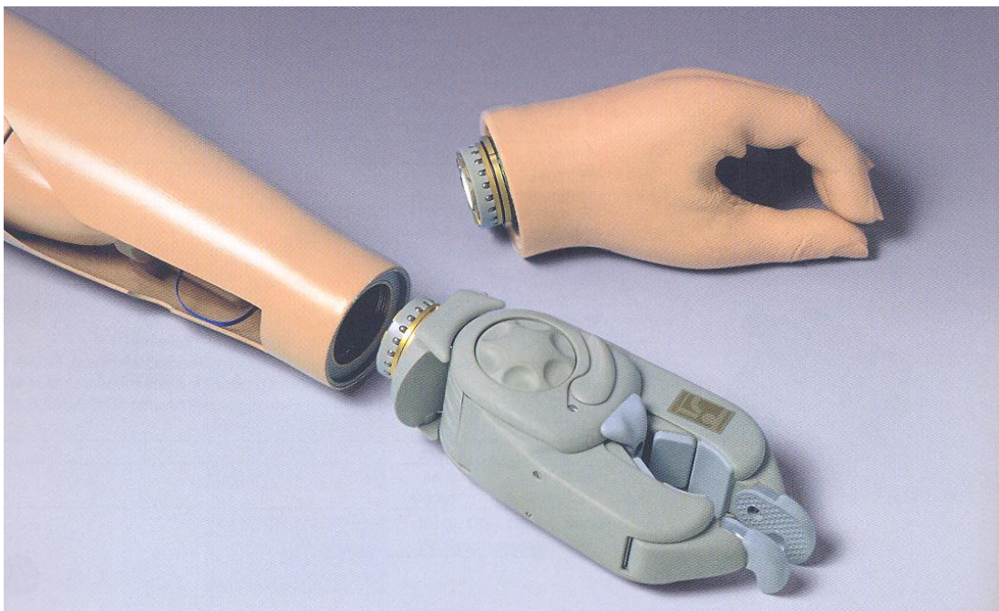
Obr. 20 Elektrická ruka a pracovní násadec [30]
